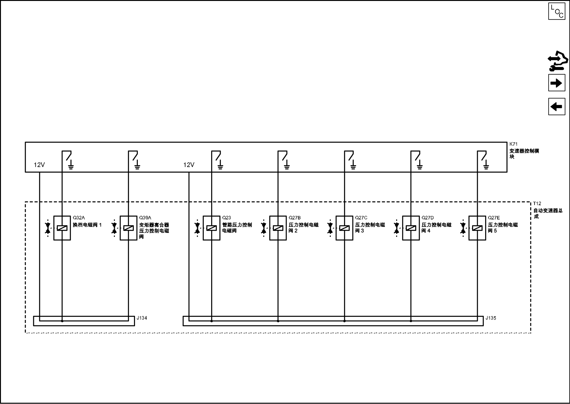
自动换档控制示意图(变速器电子阀)
