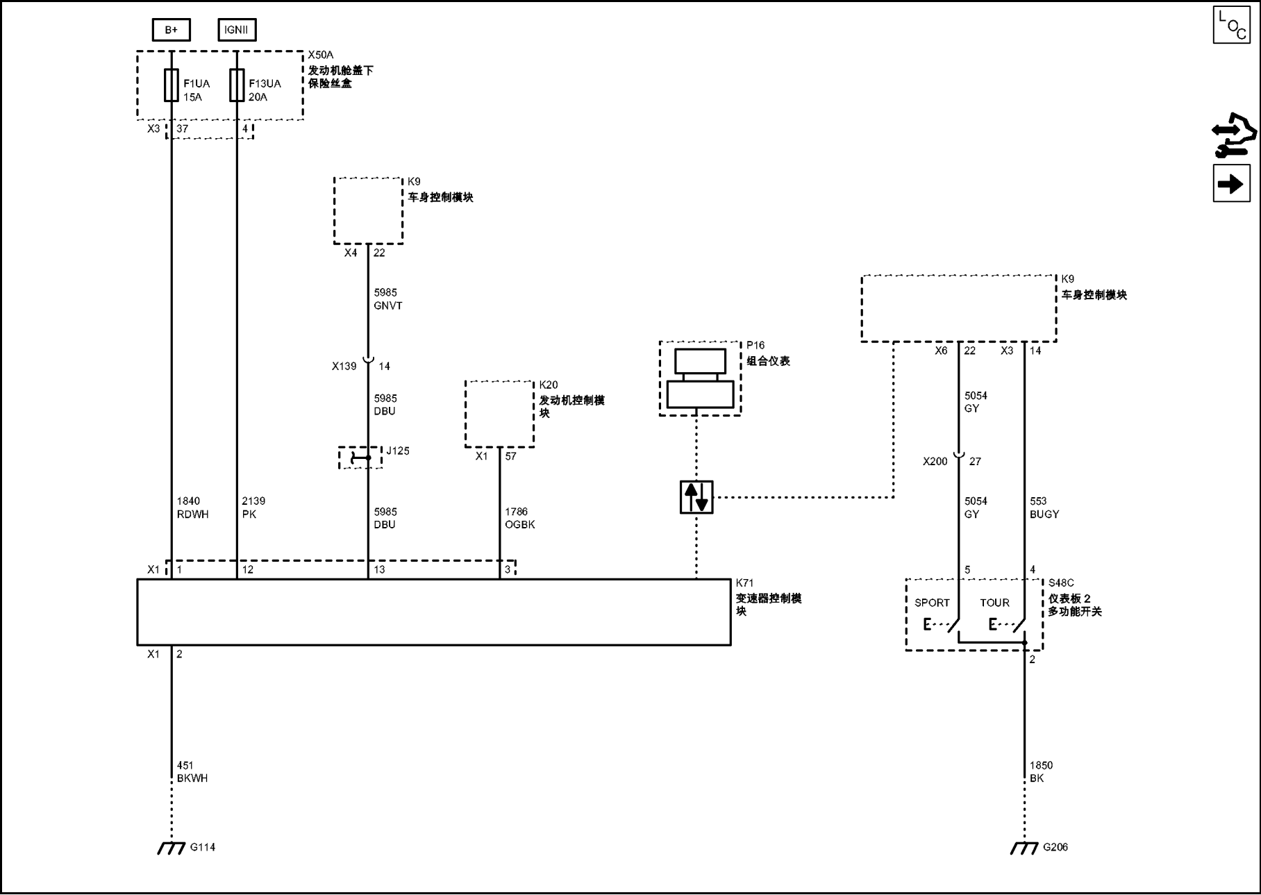
自动换档控制示意图(电源、搭铁、串行数据)
