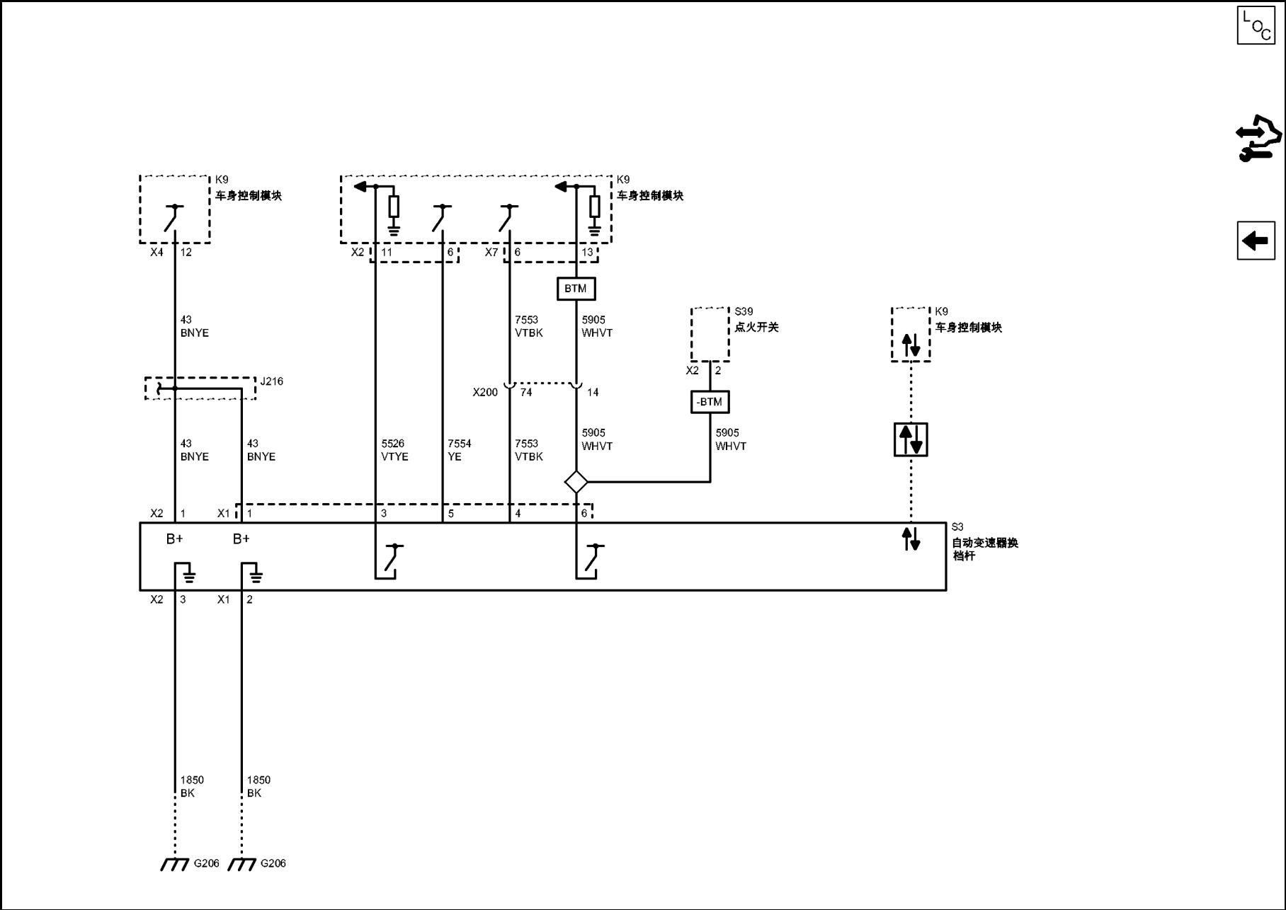
自动换挡控制示意图(换挡杆模块)
