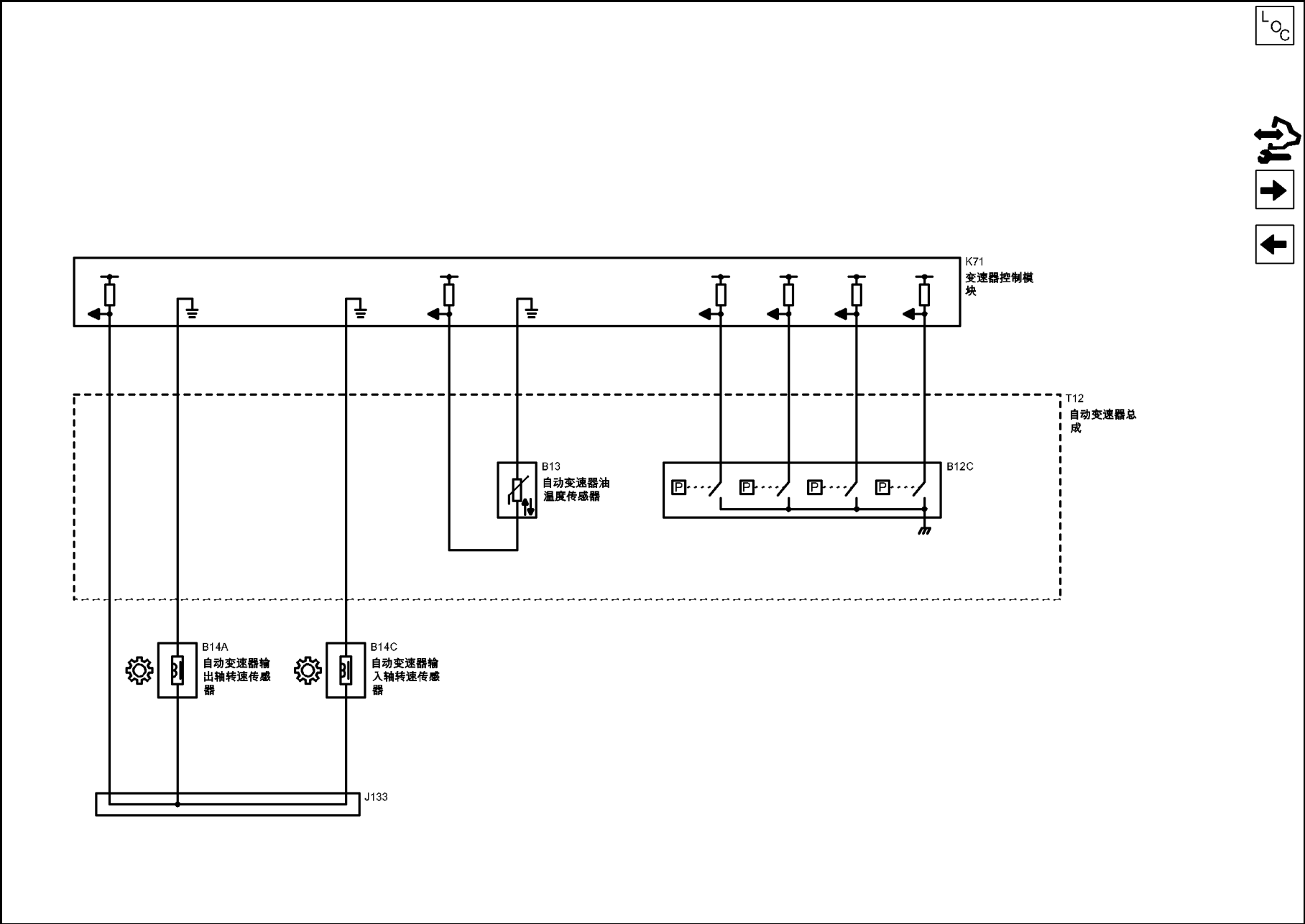
自动换档控制示意图(变速器传感器和开关)
